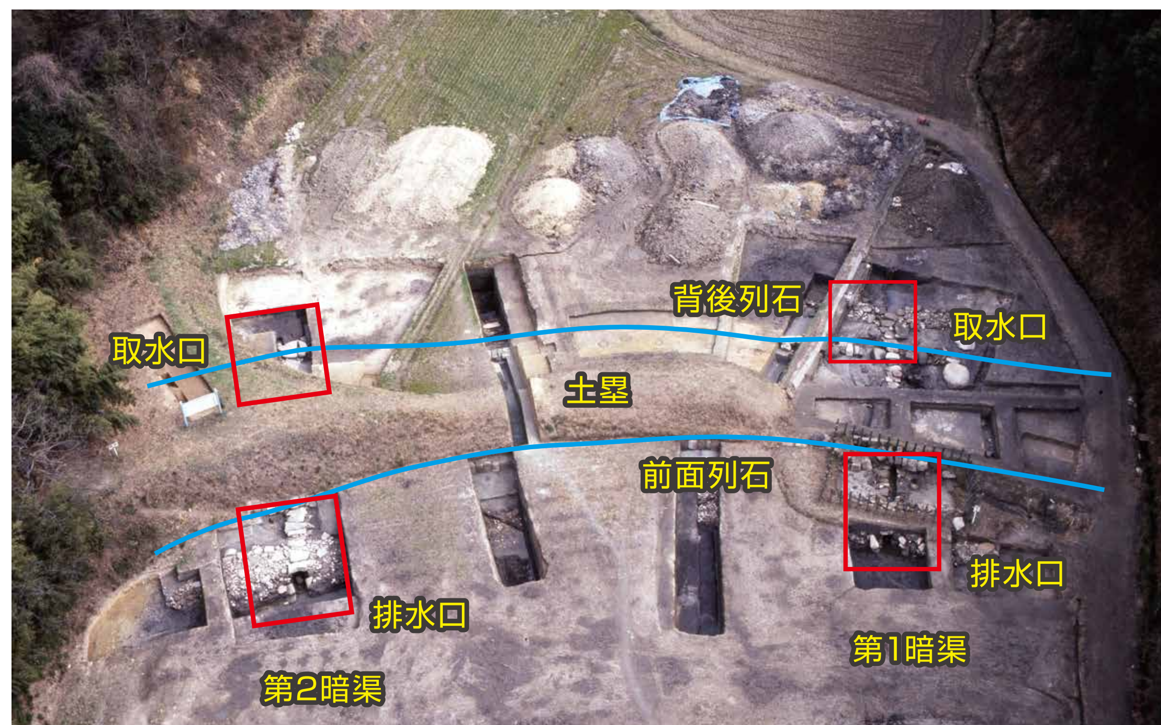
水門全景
