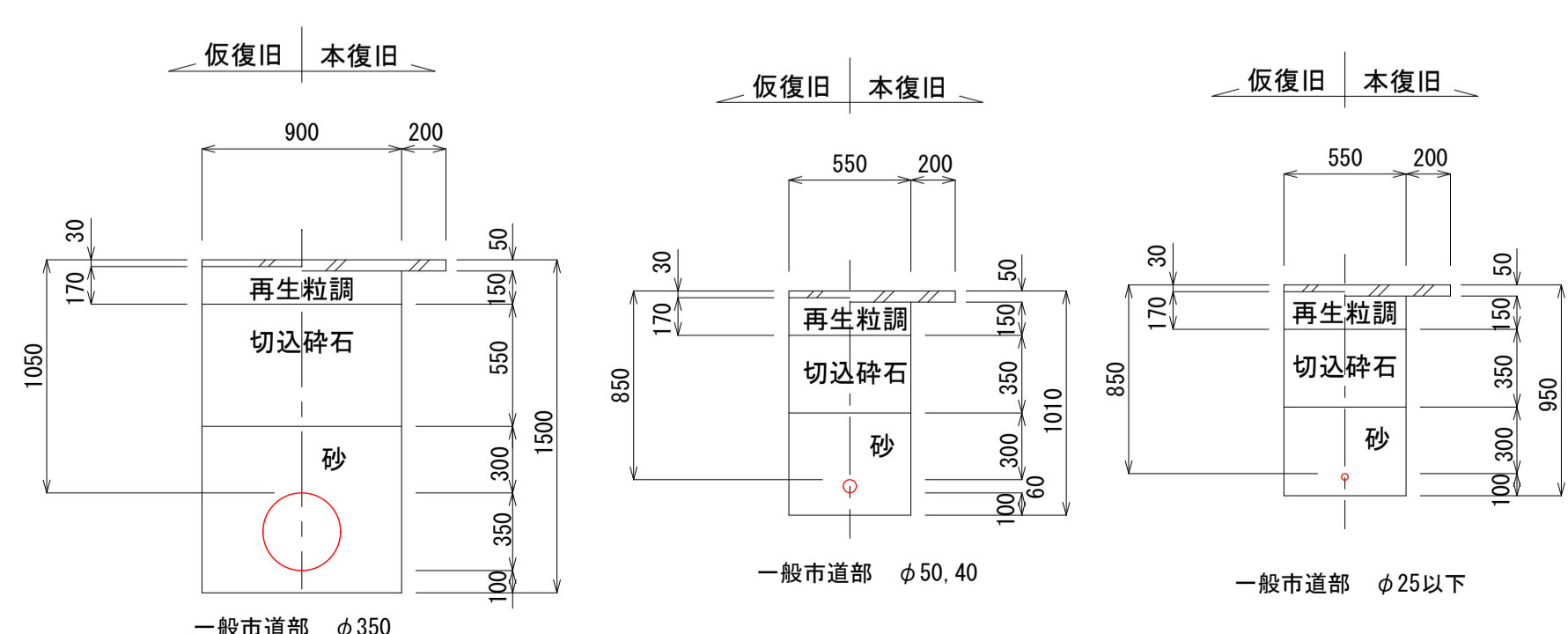
標準床掘路面復旧図 (S=1/30)
