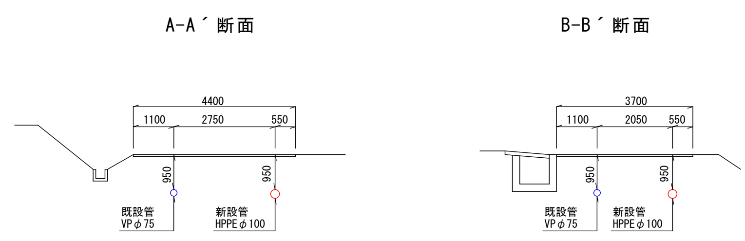
横断面図 (S=1/100)
