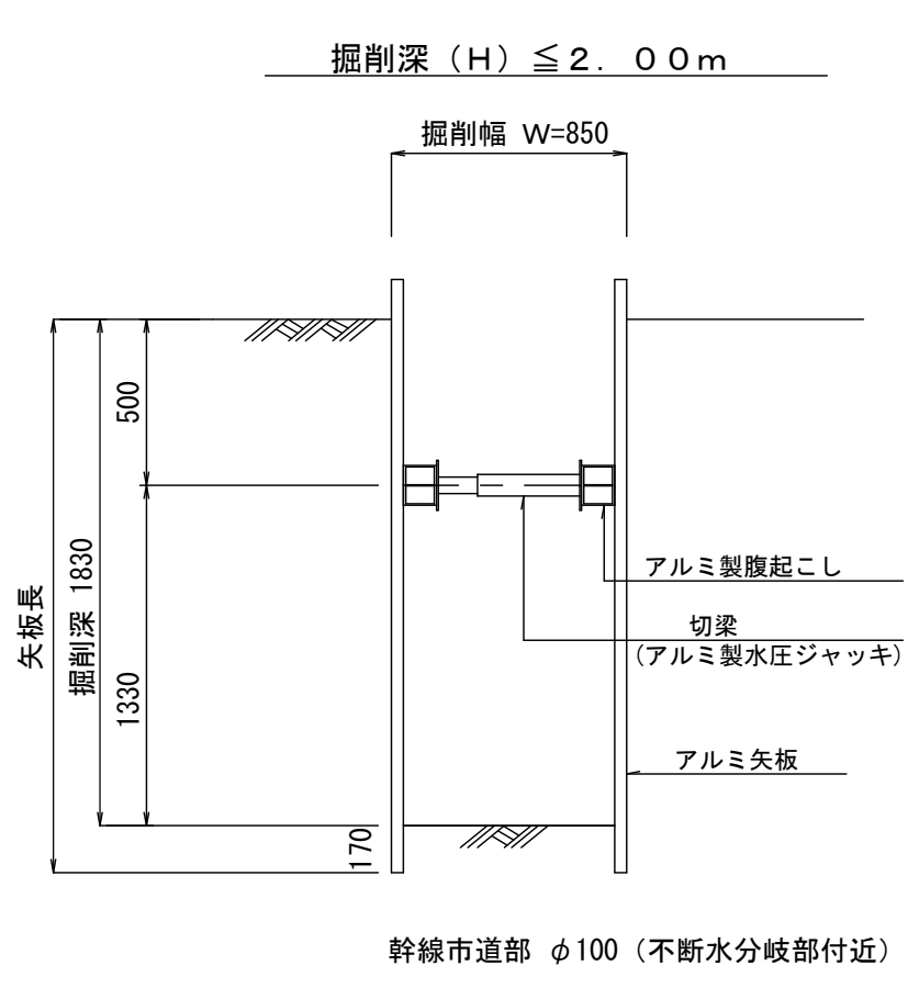
土留工標準図 (S=1:30)
