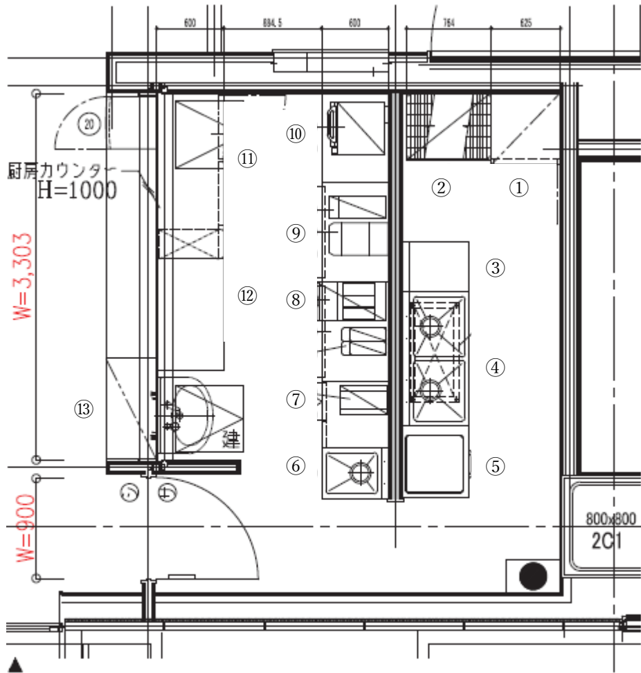
2階 厨房平面図 S=1/30
